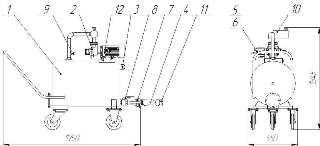
Установка вакуумная для откачки подтоварной воды
